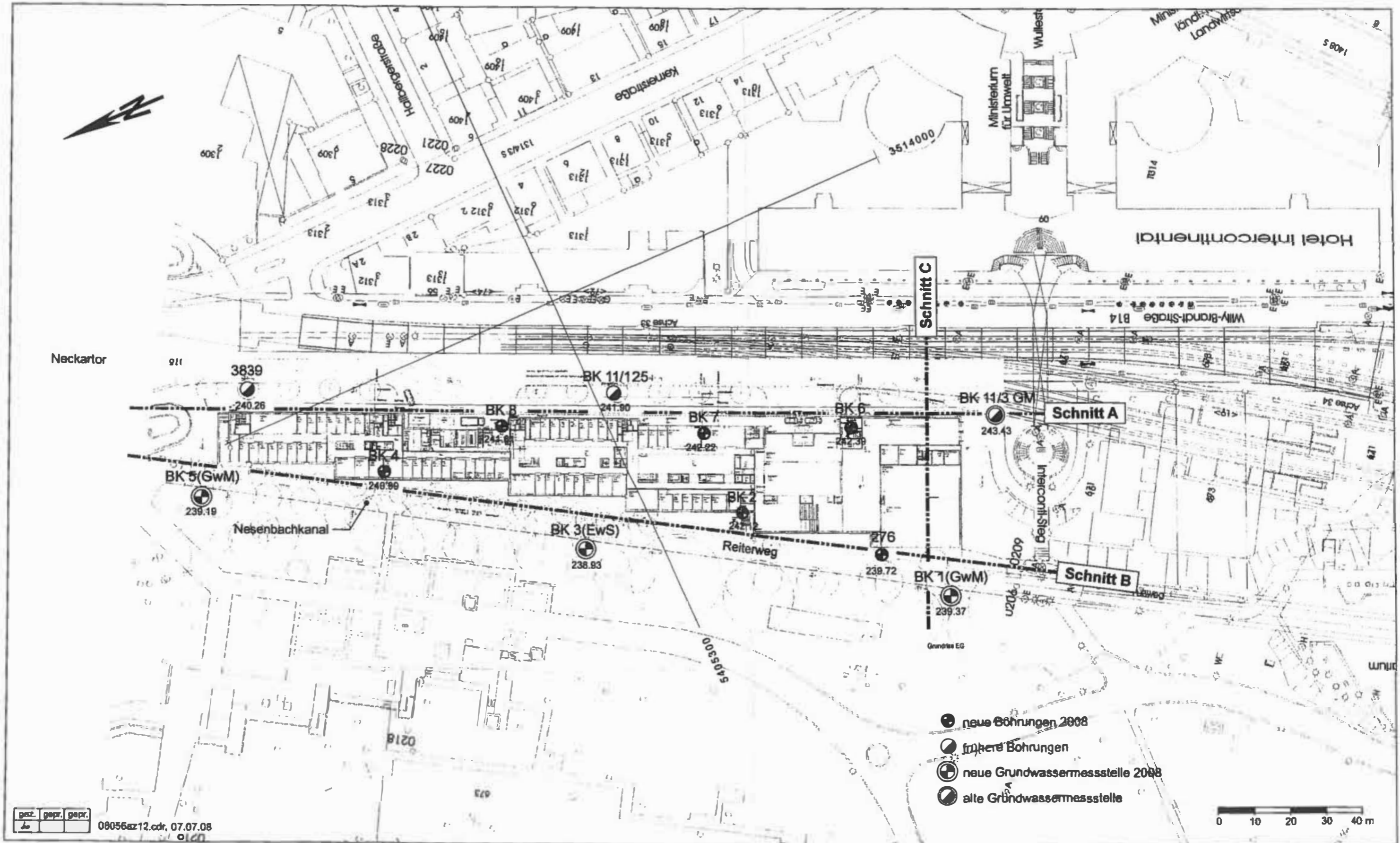
Lageplan mit Lage der Erkundungspunkte und Verlauf der geologischen Geländeschnitte
