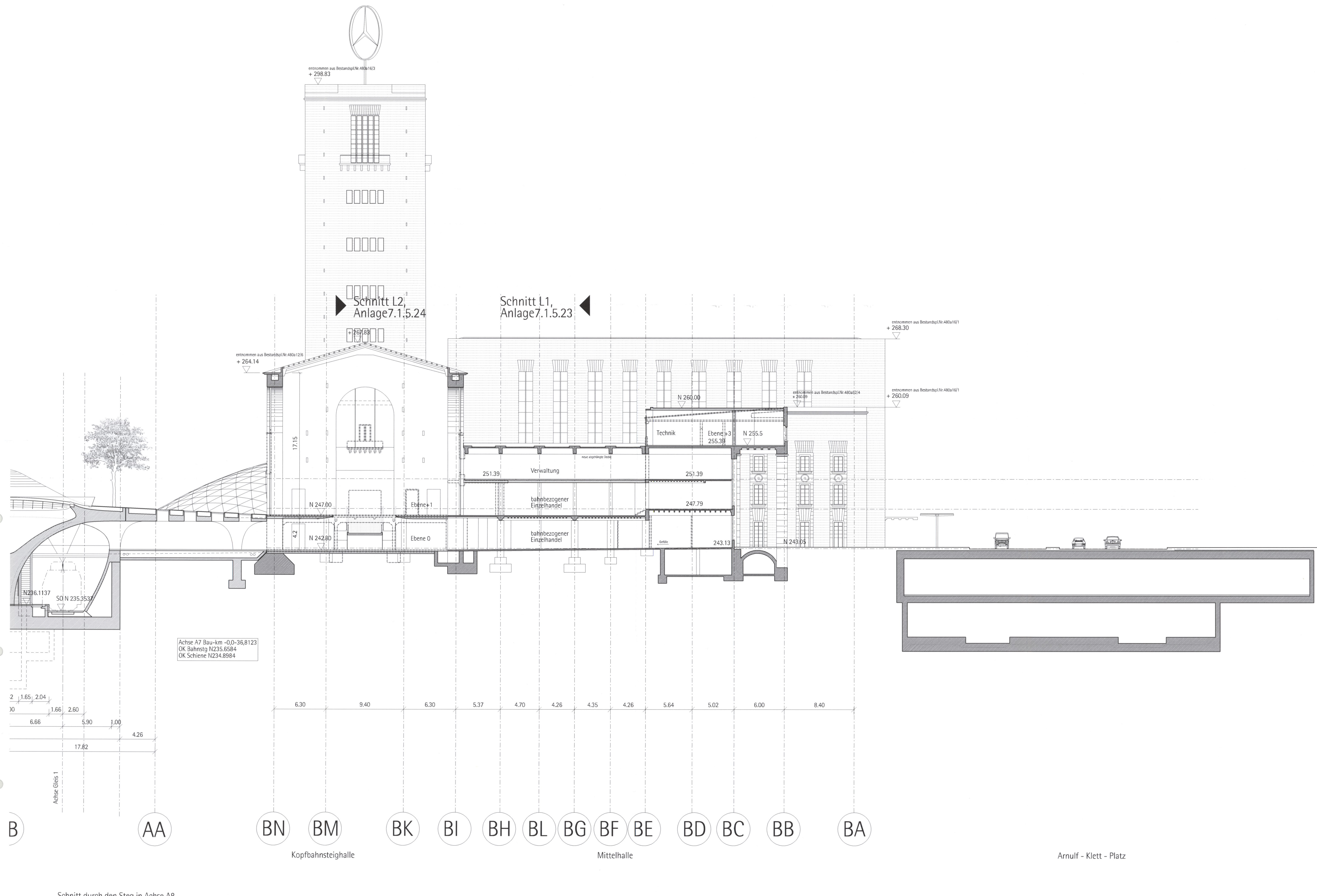
Schnitt durch den Steg in Achse A8
